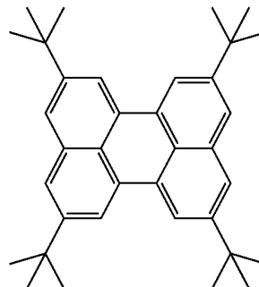
Tetra t-butyl perylene
